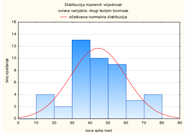
Slika 3- Distribucija mjerenih vrijednosti biomase tj korijena biomase brdskog područja
