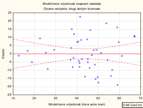
Slika 3- Prikaz rezultata modeliranih vrijednosti nasuprot ostataka modela brdskog područja
