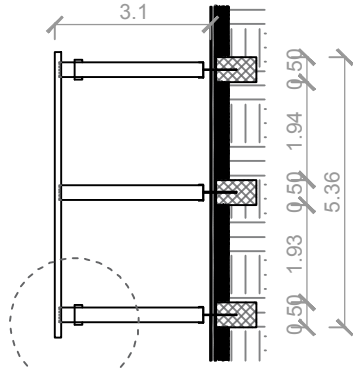
DETALJ 3
