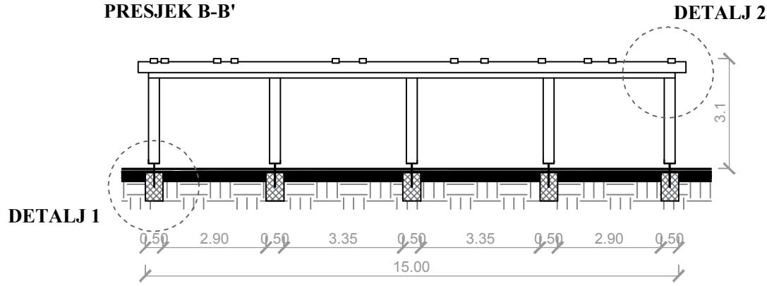
PRESJEK B-B
