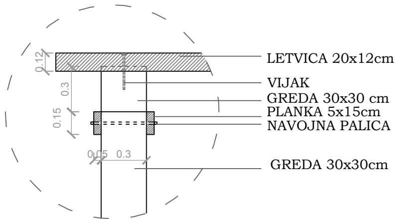
DETALJ 3-BOČNI SPOJ NA GLAVNE STUPOVE 1:25
