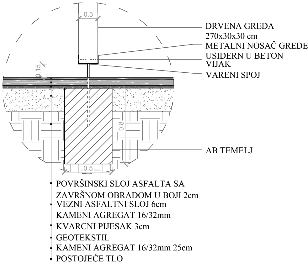
DETALJ 1- SIDRENJE STUPA PERGOLE 1:25
