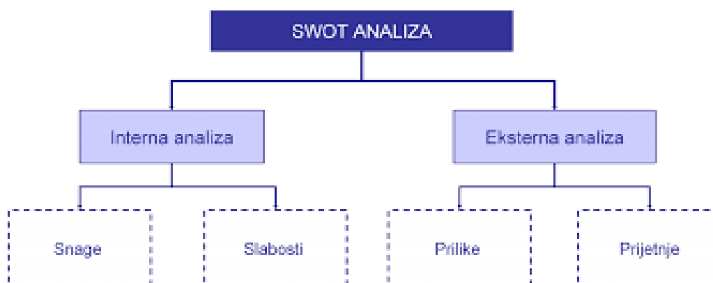
Slika 2. Shema SWOT-a
