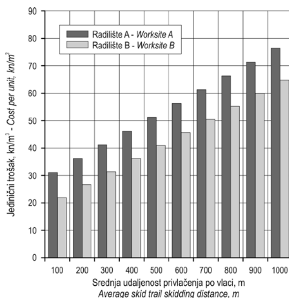
Slika 3. Ovisnost jediničnoga troška o srednjoj udaljenosti privlačenja za skider Ecotrac 120V
