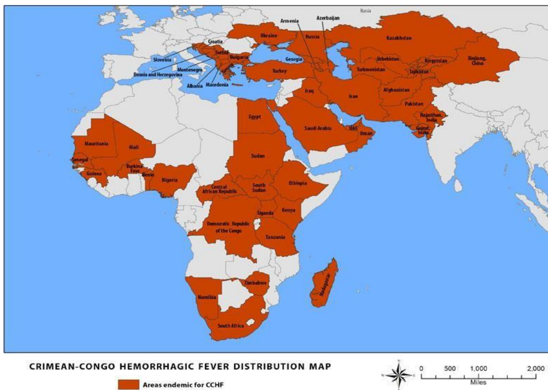
Slika 14. Karta distribucije krimsko - kongoanske groznice (Izvor: https://www.cdc.gov/ )
