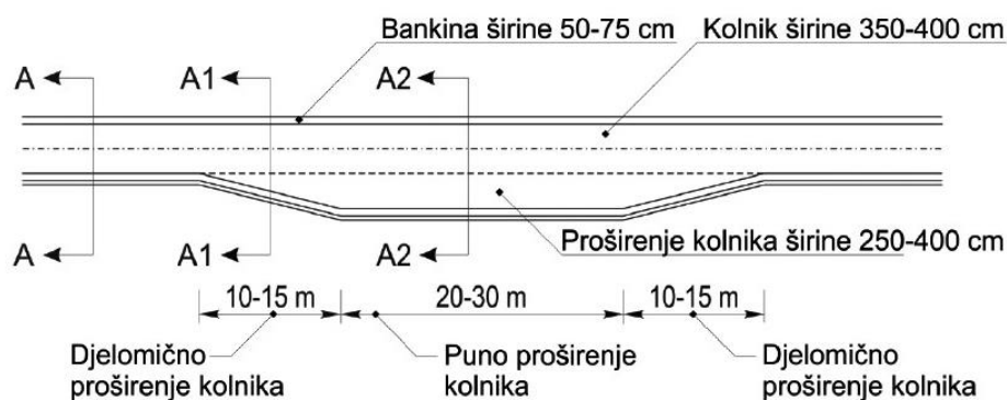
Slika 5. Detalj mimoilaznice u mjerilu M = 1:500 (autor: Pentek, T. 2018.)
