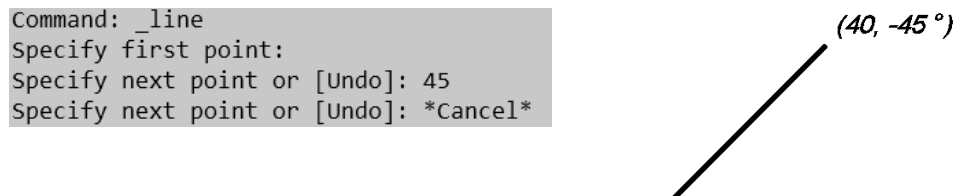
Slika 7.50 Primjer crtanja crta unosom polarnih koordinata
