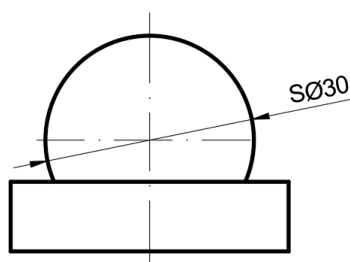
Slika 4.21 Kotiranje kugle
