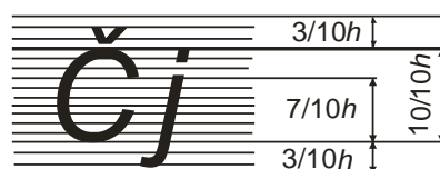
Slika 2.3 Dimenzije značajki tehničkoga pisma
