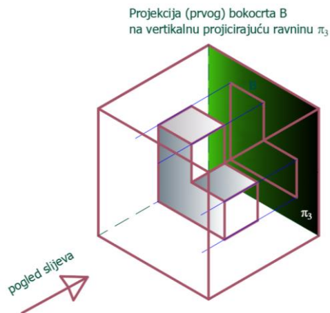
Slika 3.7 Projekcija bokocrtu
