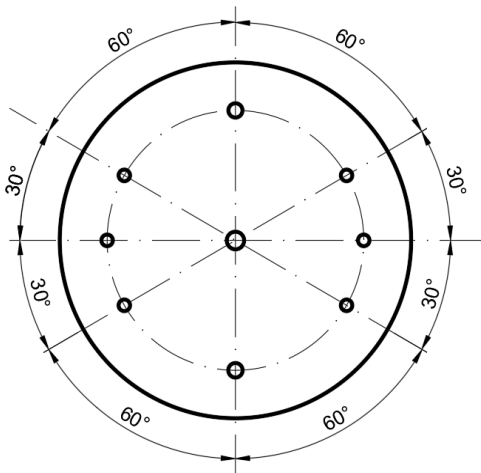
Slika 4.5 Kotiranje kutova
