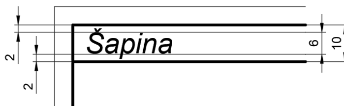
Slika 2.4 Primjer pisanja u zaglavlju s razmakom između zaglavlja i slova
