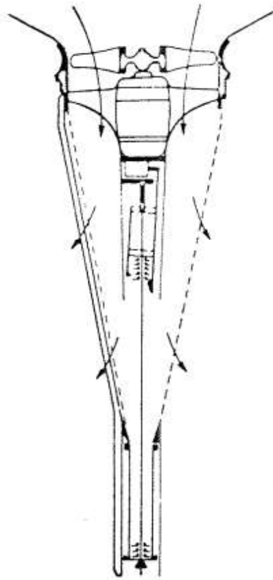
SLIKA 13. Ekshaustor
