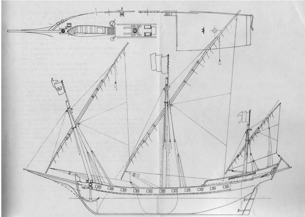
Slika 33. Skica bokeljskog šambeka (Izvor: Milošević, 1975)
