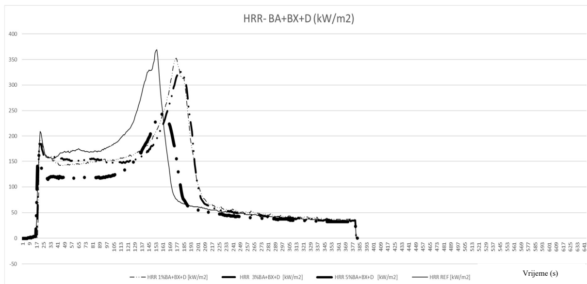
Slika 53. Grafički prikaz iznosa HRR (brzina oslobađanja topline) u \text{kW/m}^2 za vrijeme ispitivanja BA+BX+D uzoraka izmjerenih konusnim kalorimetrom
