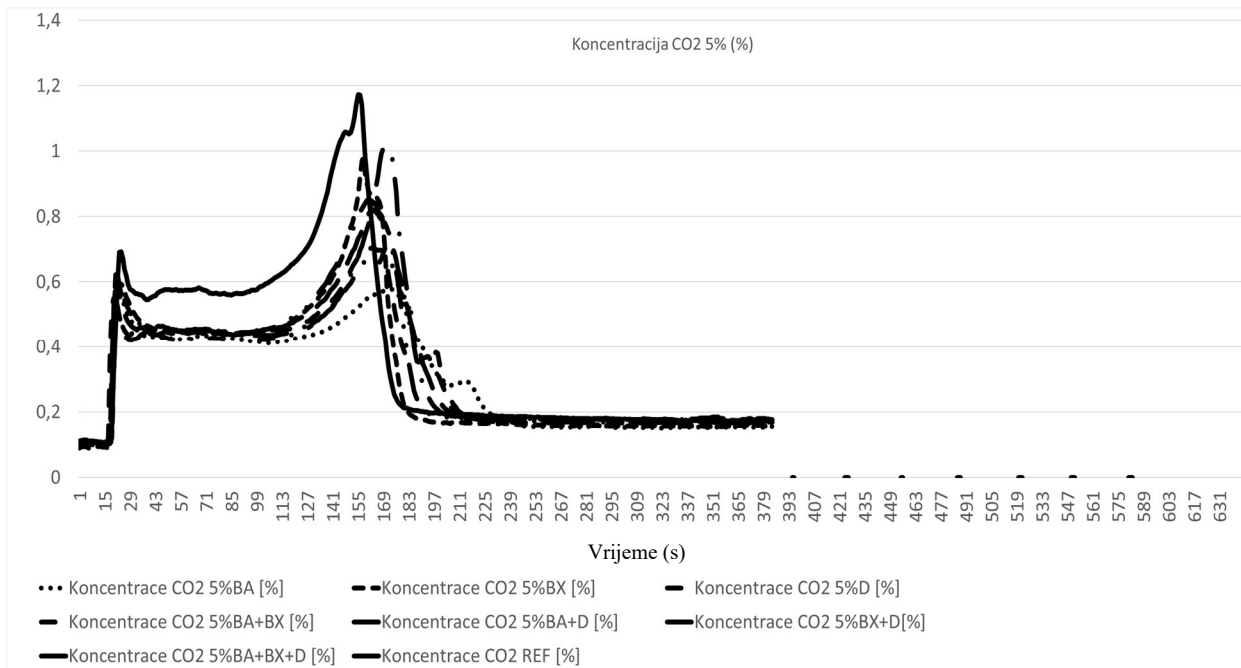
Slika 34. Grafički prikaz koncentracije CO 2 za vrijeme ispitivanja uzoraka s 5 % koncentracijom izmjerenih konusnim kalorimetrom
