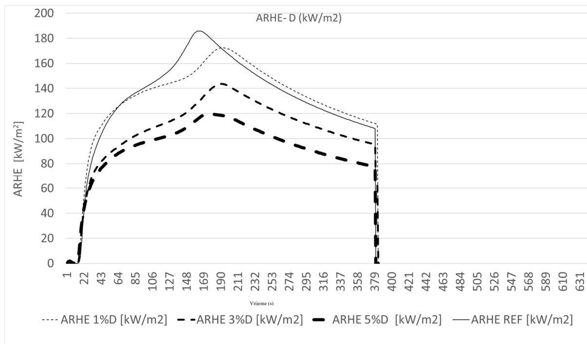
Slika 38. Grafički prikaz iznosa ARHE (prosječna brzina emisije topline) u kW/m 2 za vrijeme ispitivanja D uzoraka izmjenjenih konusnim kalorimetrom
