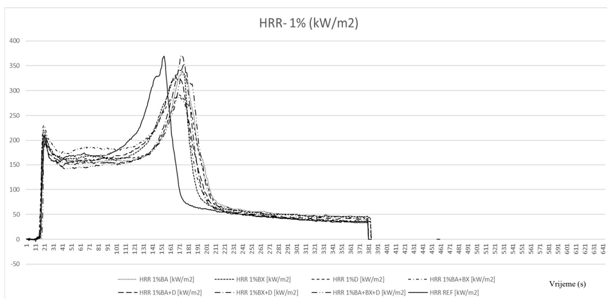
Slika 54. Grafički prikaz iznosa HRR (brzina oslobađanja topline) u \text{kW/m}^2 za vrijeme ispitivanja uzoraka s 1 % koncentracijom izmjerenih konusnim kalorimetrom
