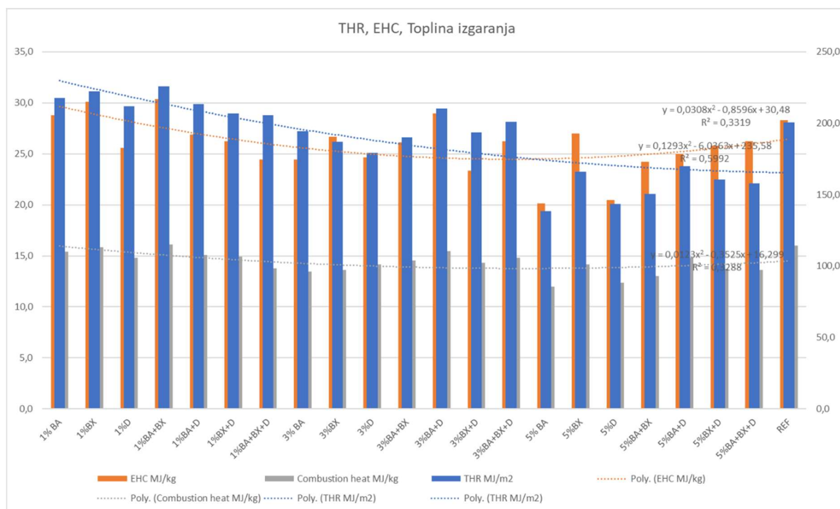
Slika 23. Grafički prikaz trenda vrijednosti EHC-a, THR-a i topline izgaranja
