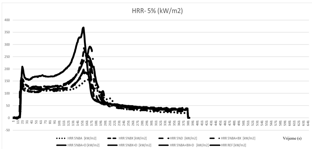
Slika 56. Grafički prikaz iznosa HRR (brzina oslobađanja topline) u \text{kW/m}^2 za vrijeme ispitivanja uzoraka s 5 % koncentracijom izmjerenih konusnim kalorimetrom
