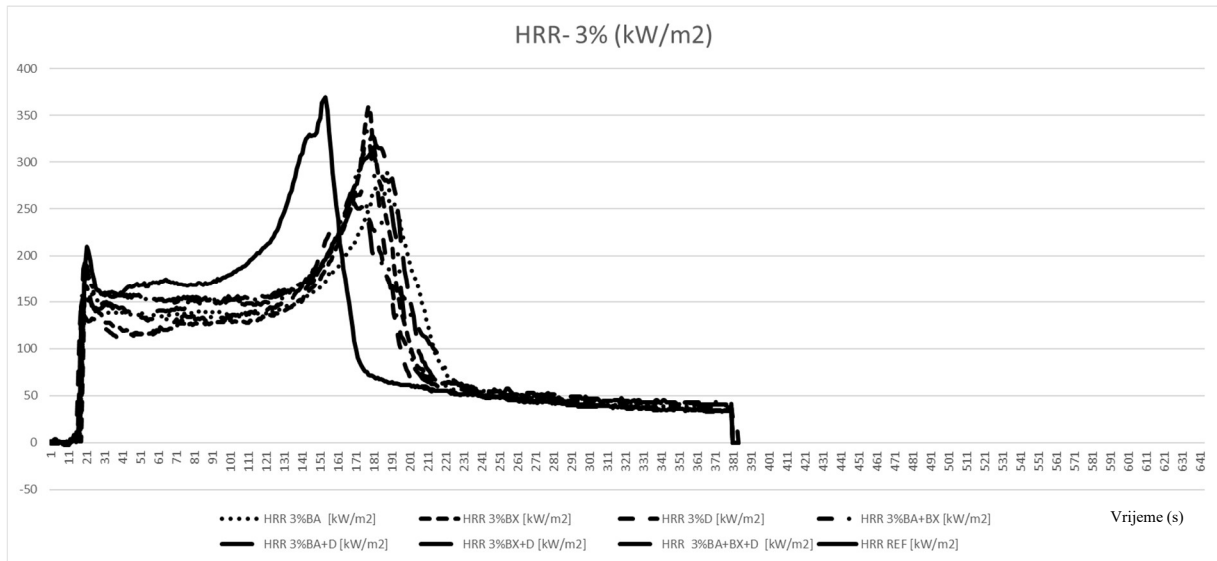
Slika 55. Grafički prikaz iznosa HRR (brzina oslobađanja topline) u \text{kW/m}^2 za vrijeme ispitivanja uzoraka s 3 % koncentracijom izmjerenih konusnim kalorimetrom
