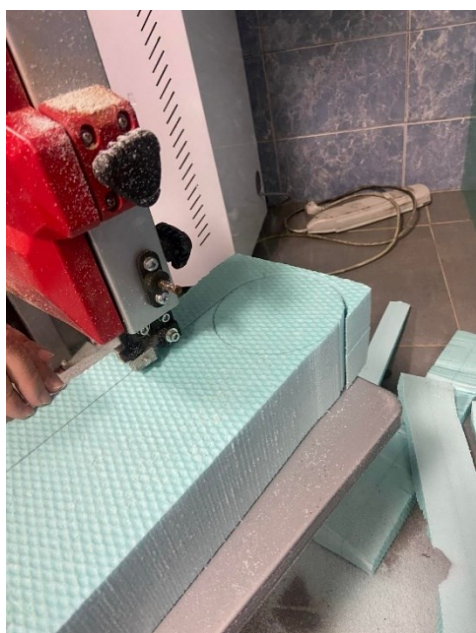
Slika 19. Prikaz piljenja šablone na tračnoj pili.
