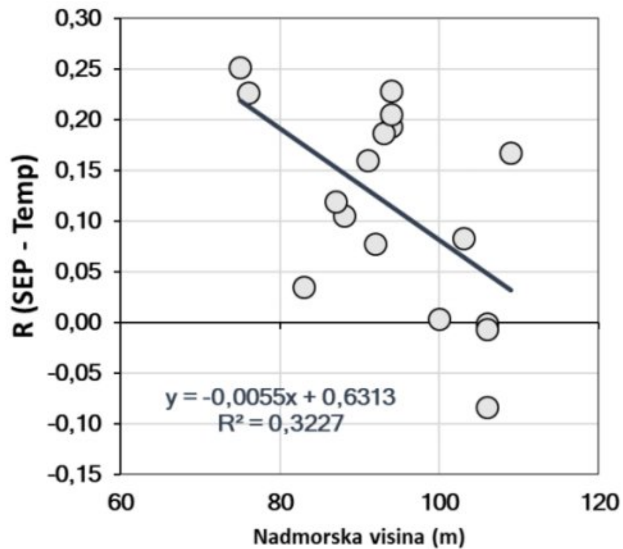
Slika 21. Linearna regresija između korelacija s temperaturom zraka u rujnu (SEP) obzirom na nadmorsku visinu lokaliteta.
