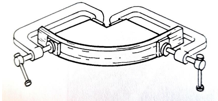
Slika 15. Savijanje između muškog i ženskog kalupa (Taylor,2001)
