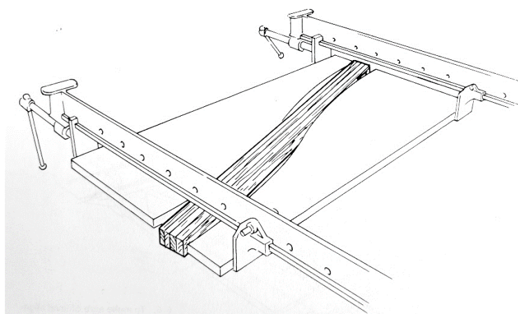
Slika 16. Savijanje u oblik slova S (Taylor,2001)
