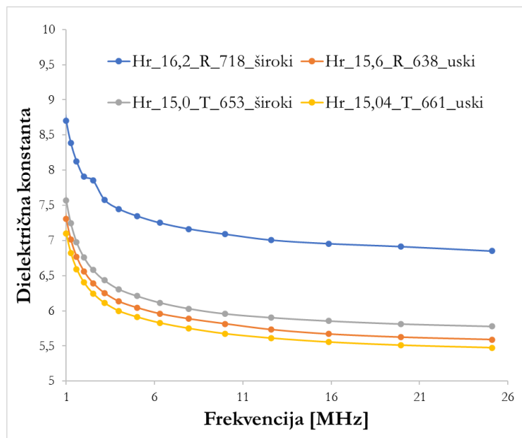
Slika 45. Dijagram ovisnosti srednje vrijednosti dielektrične konstante o frekvenciji električnog polja od 1 MHz do 25 MHz pri sadržajima vode hrastovih lamela od 15 do 16,2 %
