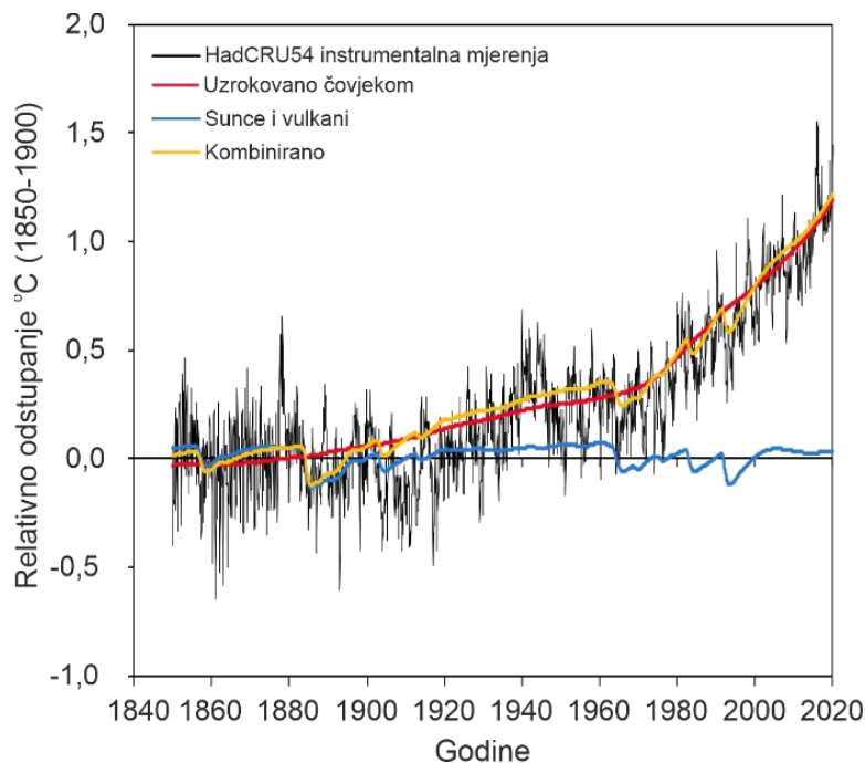
Slika 1. Indeks globalnog zatopljenja (GWI) od 1850. do 2020. godine. Antropogeni doprinos globalnom zagrijavanju prikazan crvenom bojom. Prirodni doprinos (sunce i vulkanski) u plavoj boji. Žuta linija prikazuje kombiniranu (ukupnu) promjenu temperature
