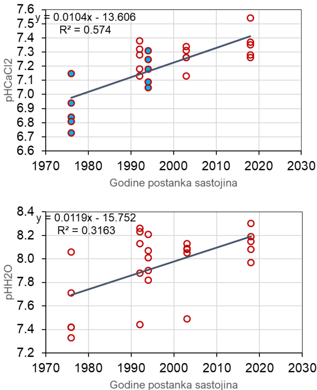
Slika 22 Ovisnost pH tla o godini postanka sastojine za sve plohe zajedno. Plavom bojom su označene kontrolne plohe.
