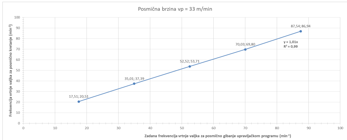
Slika 38. Ovisnost postavljene i mjerene frekvencije vrtnje
