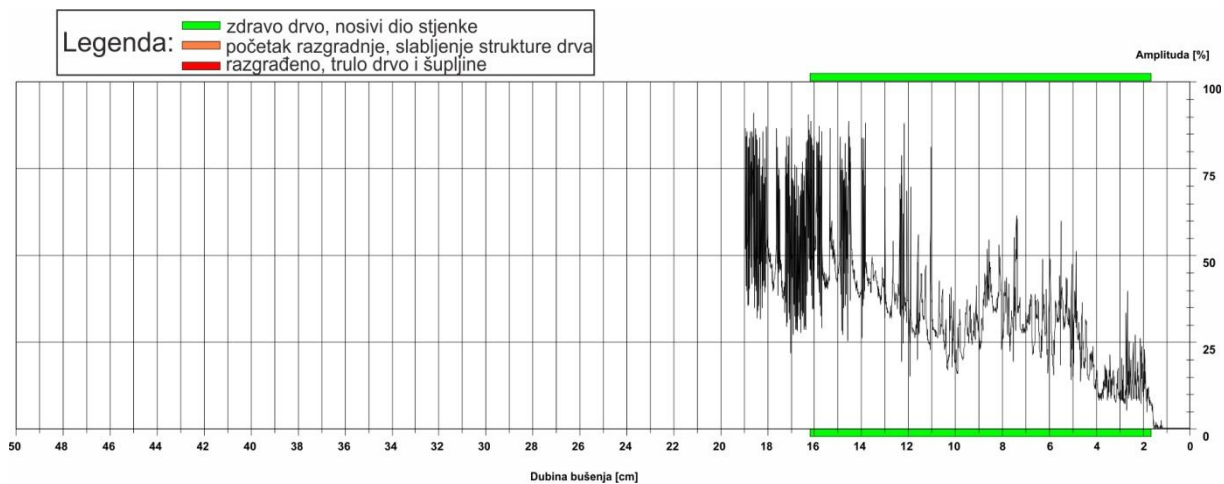
Slika 24: Rezistogram bušenja 9
