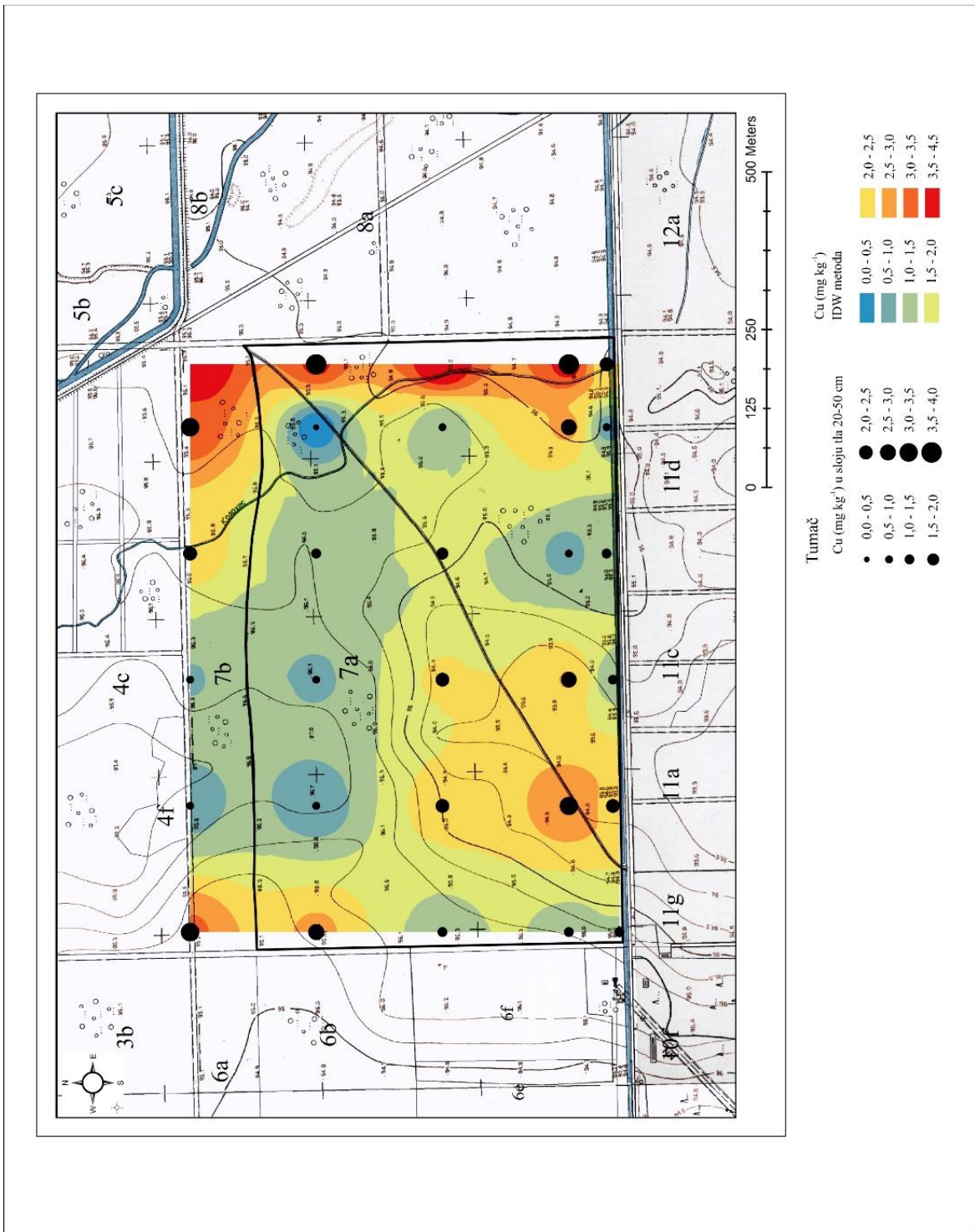
Slika 28. Prostorna distribucija bakra (mg kg -1 ) u tlu za dubinu 20-50 cm na području prašume Prašnik
