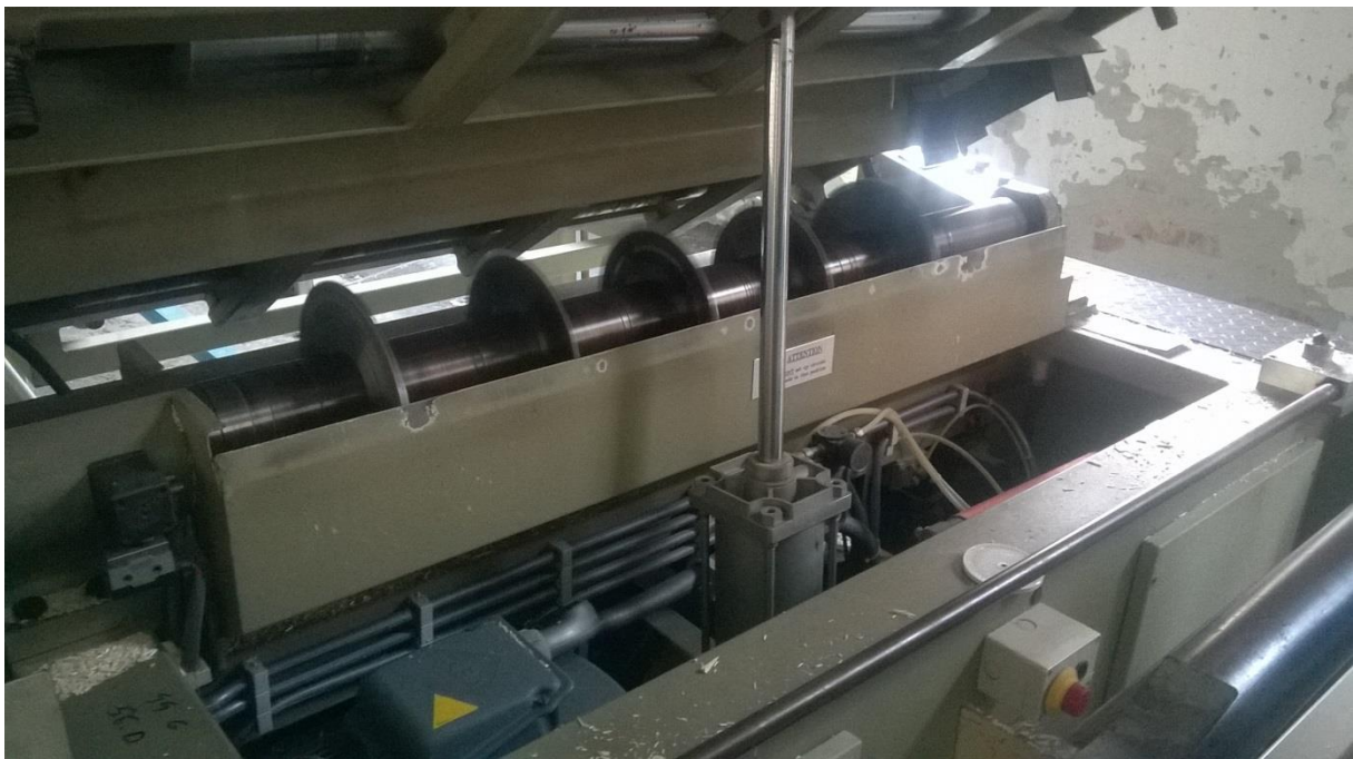
Slika 16. Pile na višelisnom cirkularu za raspiljivanje slijepljenih ploča u parketne daske.
