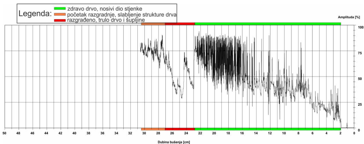
Slika 26: Rezistogram bušenja 11
