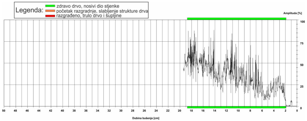
Slika 16: Rezistogram bušenja 3
