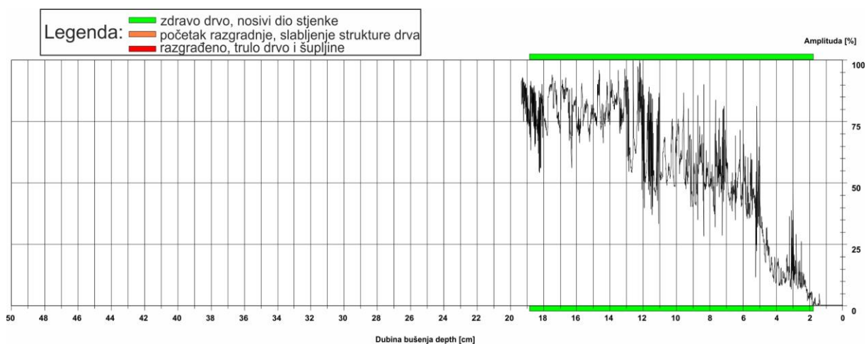
Slika 32: Rezistogram bušenja 14
