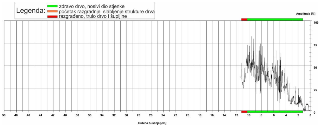
Slika 19: Rezistogram bušenja 7
