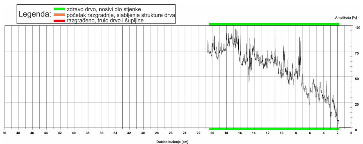
Slika 18: Rezistogram bušenja 5.1
