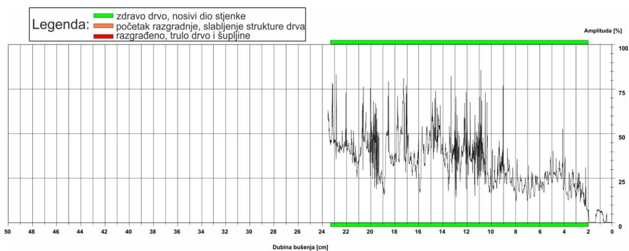
Slika 30: Rezistogram bušenja 13
