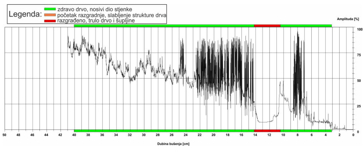
Slika 33: Rezistogram bušenja 15
