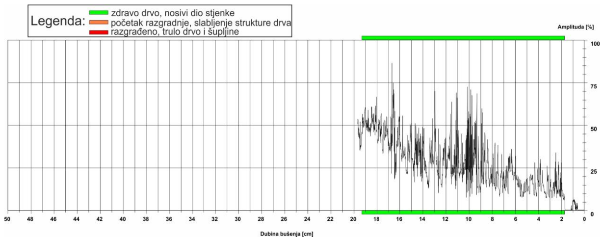
Slika 17: Rezistogram bušenja 5
