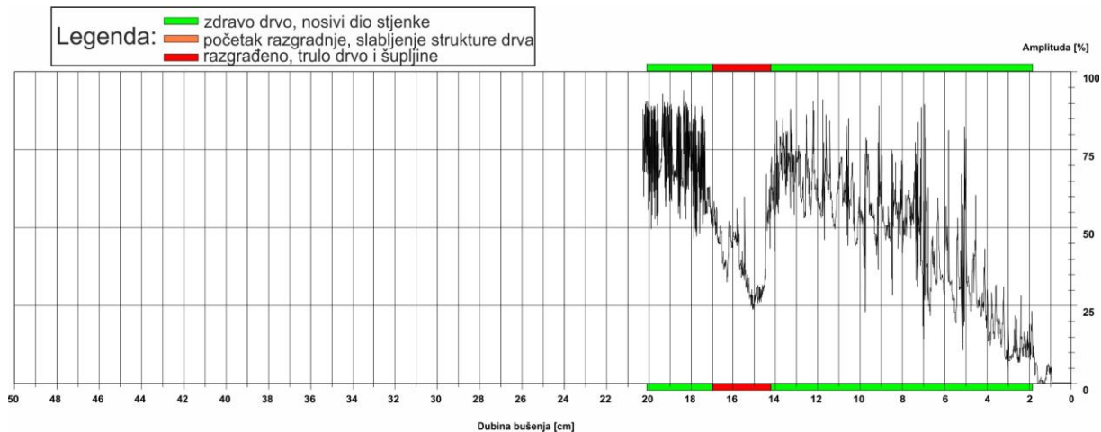
Slika 25: Rezistogram bušenja 10
