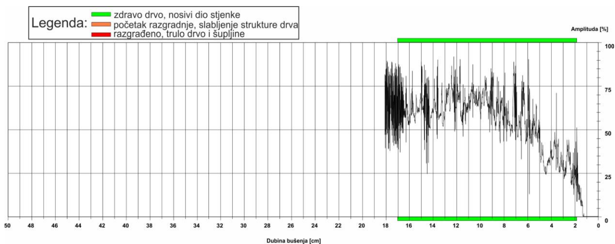
Slika 23: Rezistogram bušenja 8.1
