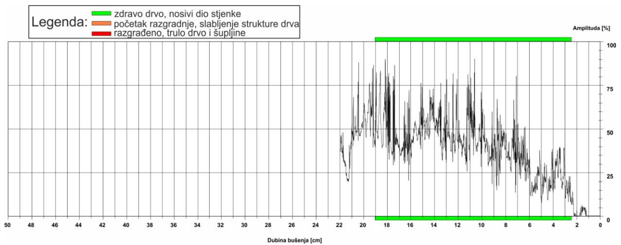
Slika 21: Rezistogram bušenja 6.1
