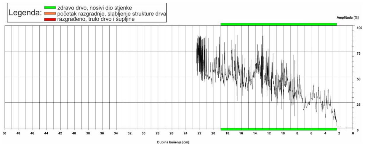
Slika 20: Rezistogram bušenja 6
