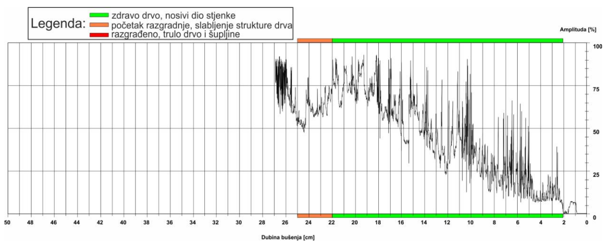
Slika 27: Rezistogram bušenja 11.1
