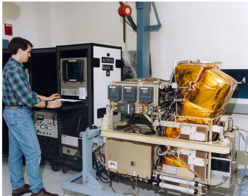
Slika 7.: AVIRIS hiperspektralni senzor ( https://www.nasa.gov/images/content/612114main_AVIRIS_checkout.jpg )
