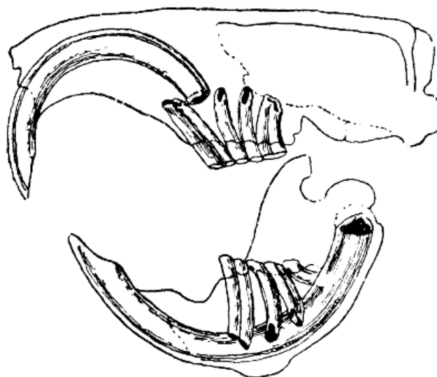
Slika 2. Lubanja glodavca
