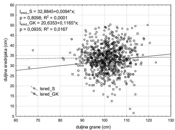
Slika 12. Ovisnost duljine srednjaka o duljini grane
