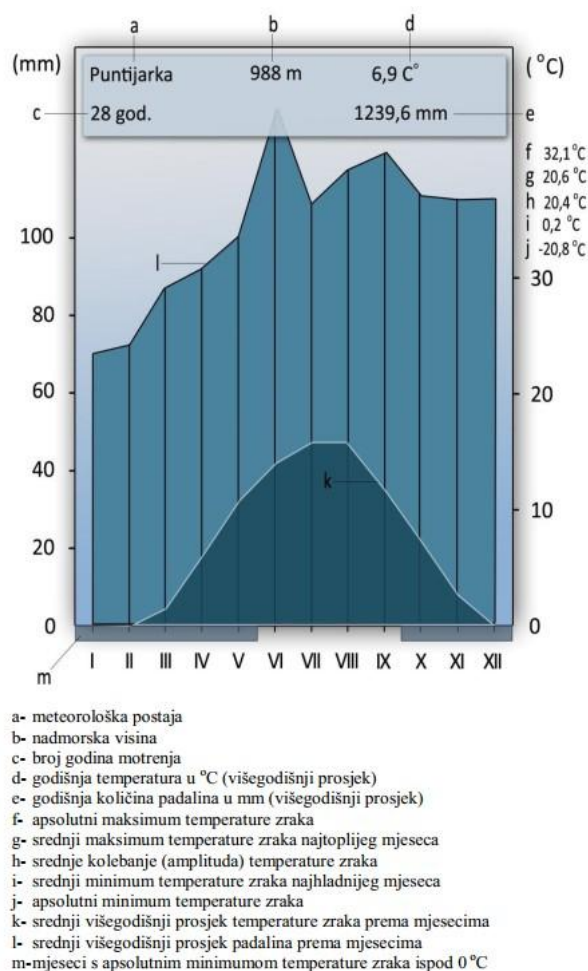
Slika 4: Walterov klimadijagram za meteorološku postaju Puntijarka,
