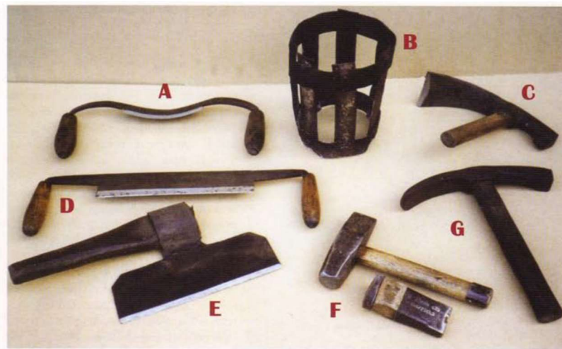
Slika 3. Osnovni ručni alat bačvara (A – nož za dubljenje, B – posuda za paljenje vatre unutar bačve, C – sjekira širočka (bradva), D – nož za ravne plohe (drawknife), E – sjekira, F i G – čekići i klin za navlačenje obruča)
