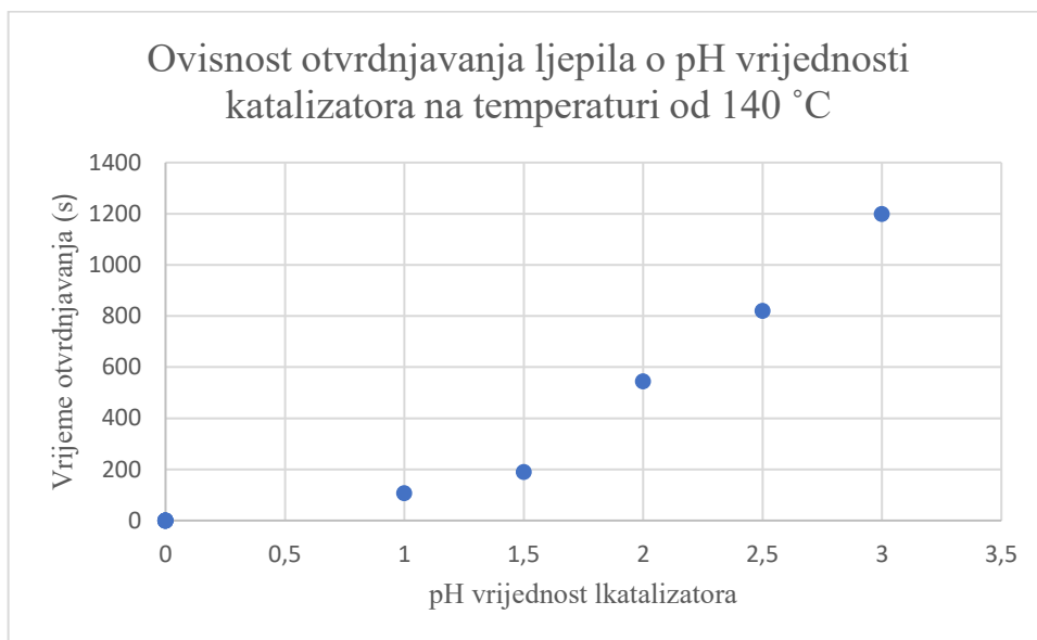
Slika 20. Ovisnost otvrdnjavanja ljepljiva o pH vrijednosti katalizatora na temperaturi od 140 °C (UF smola)
