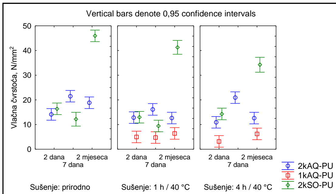
Slika 29. Utjecaj vrste, trajanje sušenja i trajanje kondicioniranja na vlačnu čvrstoću lakova na bazi poliuretana (2kAQ-PU: dvokomponentni vodeni lak, 1kAQ-PU: jednodokomponentni vodeni lak, 2kSO-PU: dvokomponentni otapalni lak)
