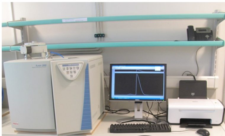
Slika 7. CHNSO/O Flash 112 tvrtke Thermo-scientific.
