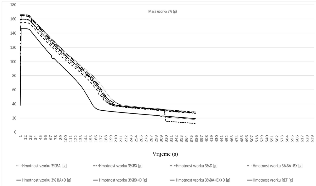
Slika 29. Grafički prikaz gubitka mase za vrijeme ispitivanja uzoraka s 3 % koncentracijom izmjerenih konusnim kalorimetrom
