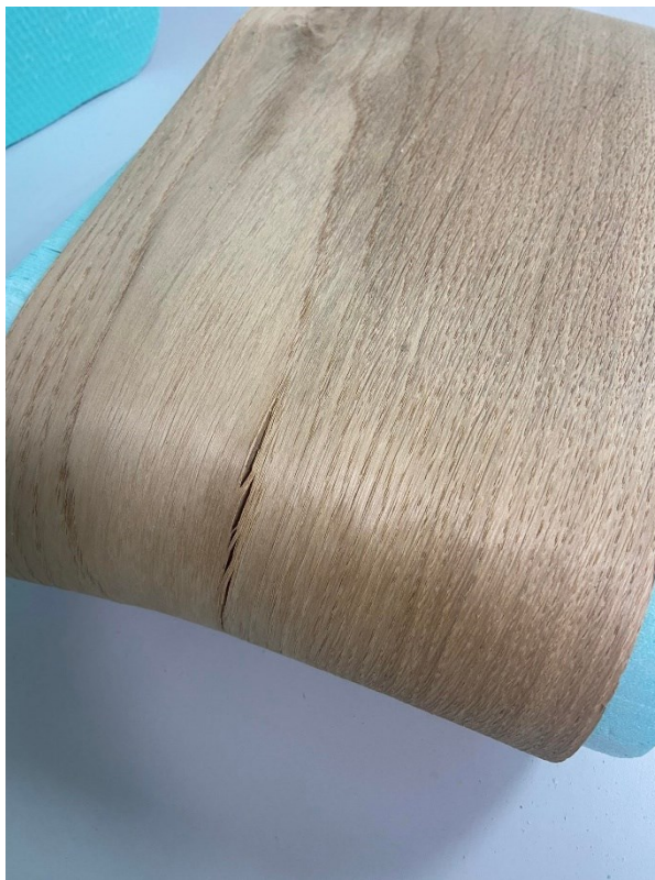
Slika 21. Prikaz pukotine nastale sušenjem (zatezanjem) furnira.
