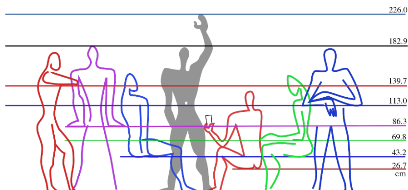
Slika 65. „Modulor“
