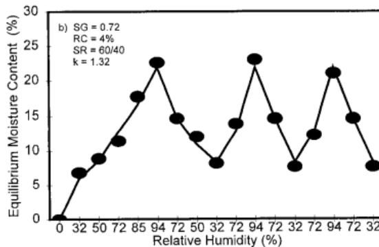
Slika 2b. Usporedba izmjerenih i predviđenih sorpcijskih izoterma pod cikličkim uvjetima za troslojne ploče
