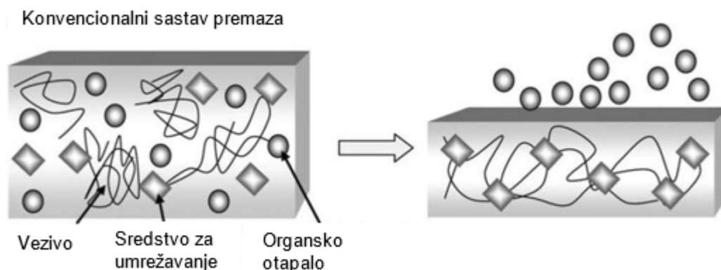
Slika 1. Konvencionalni sastav premaz (Glöckner i drugi, 2008)
