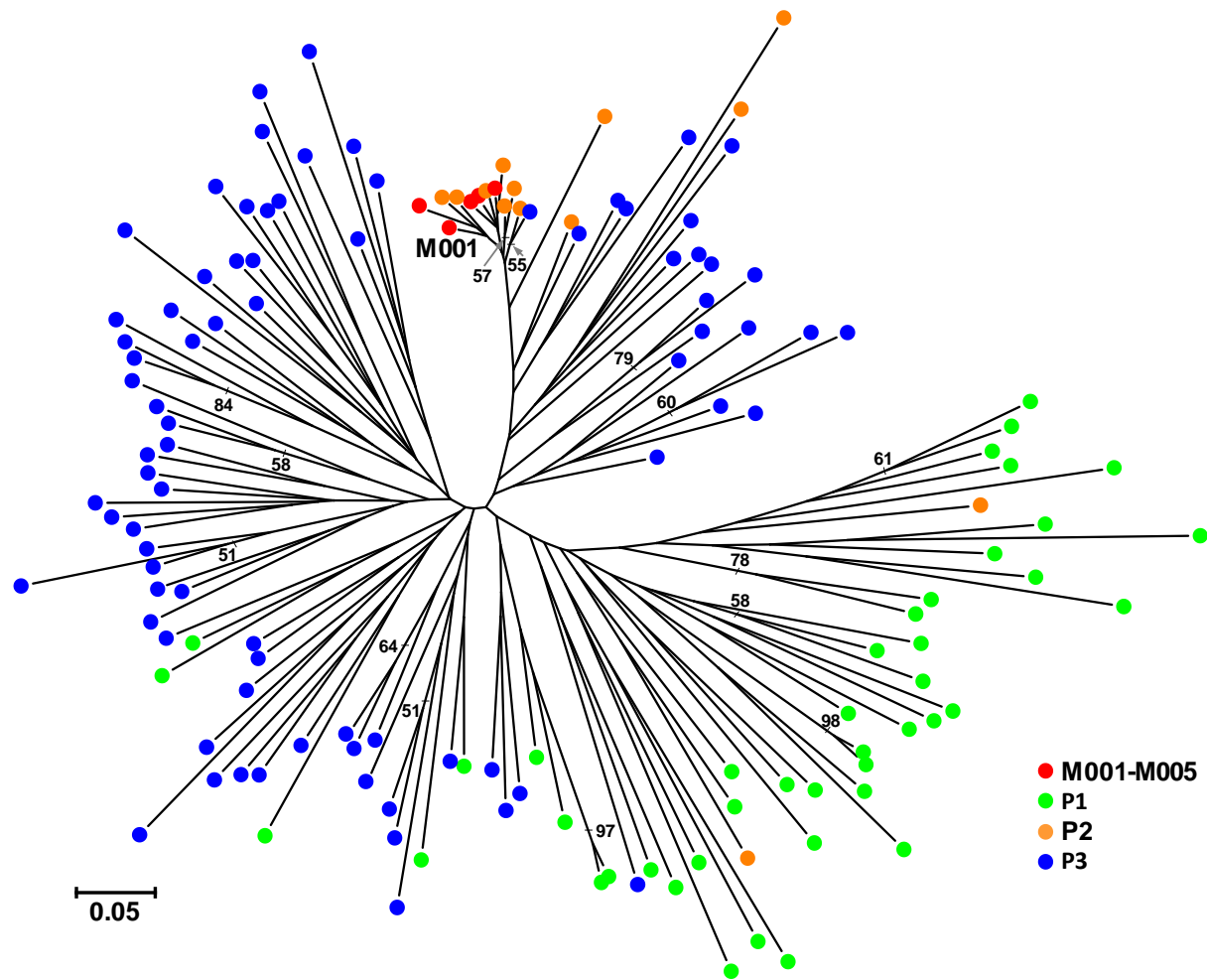
Slika 7. Nezakorijenjeno stablo nastalo na temelju podataka o raznolikosti mikrosatelitnih biljega 141 jedinice multilokusnih genotipova kestena analiziranih u ovome istraživanju. Marunska (klonalna) grupa M001-M005, kao i populacija kojoj pojedina jedinka pripada (P1, P2, P3) naznačene su na svakoj grani stabla. Brojevi iznad grana predstavljaju pripadajuće bootstrap vrijednosti iznad 50 %, u 1000 pseudoreplikacija.
