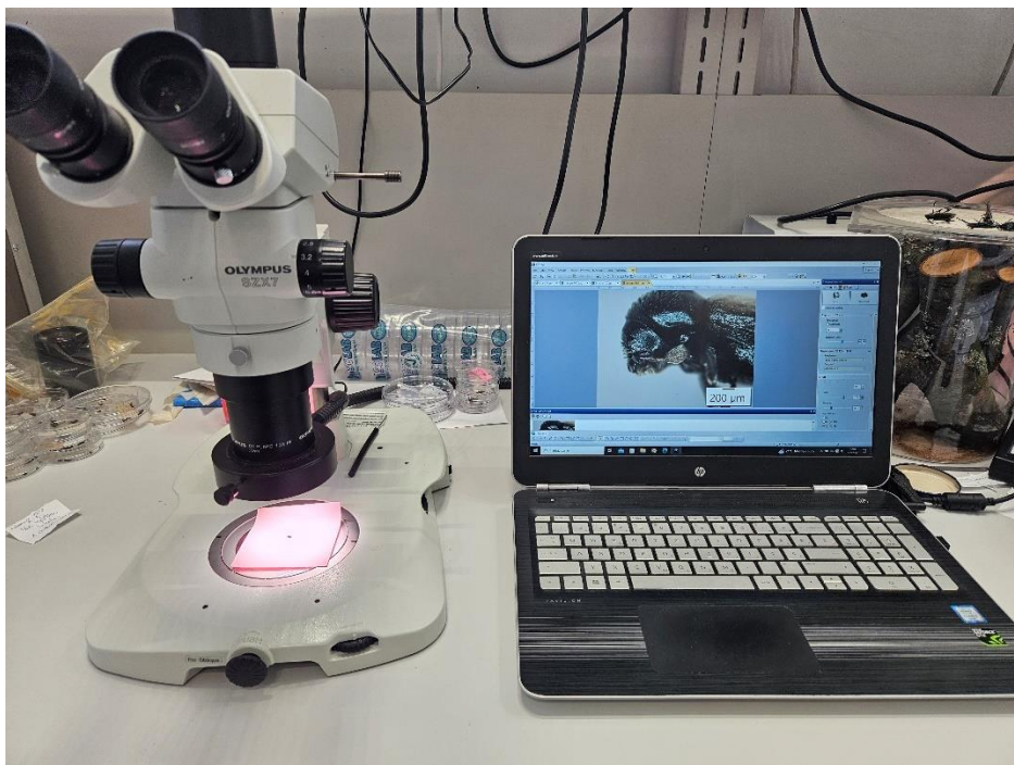
Slika 16. Determinacija kolateralnih ulova pomoću binokularne lupe (Olympus SZX7 + EP50)
