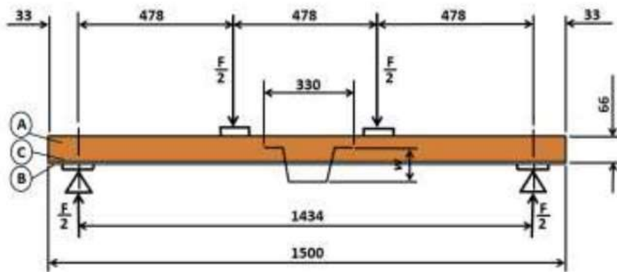
Slika 3. Prikaz opterećenja uzorka (Šedivka i ostali, 2015.)
