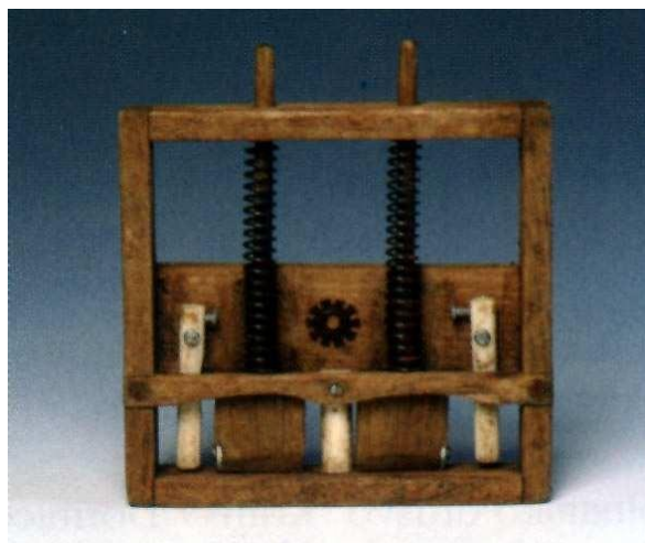
Slika 19. Selektivna puholovka, izum Marijana Zavodnika (snimio: Tomislav Šporer)
