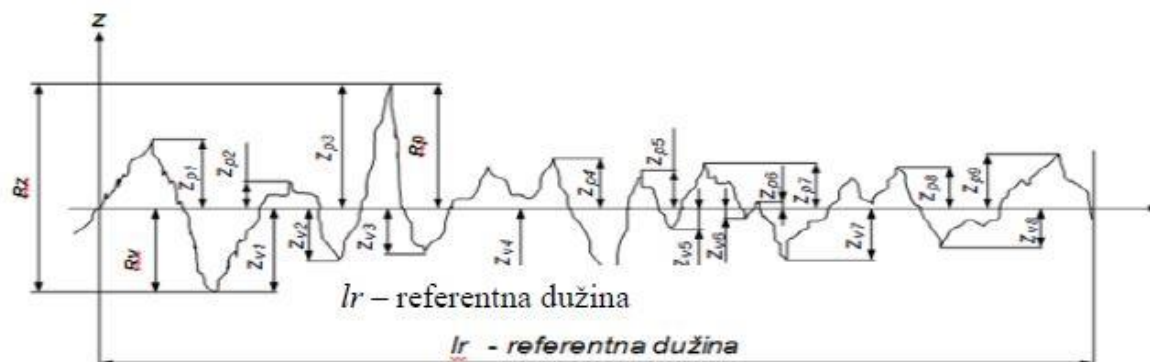
Graf 4. Grafički prikaz parametra hrapavosti R_z (Runje, 2014.)
