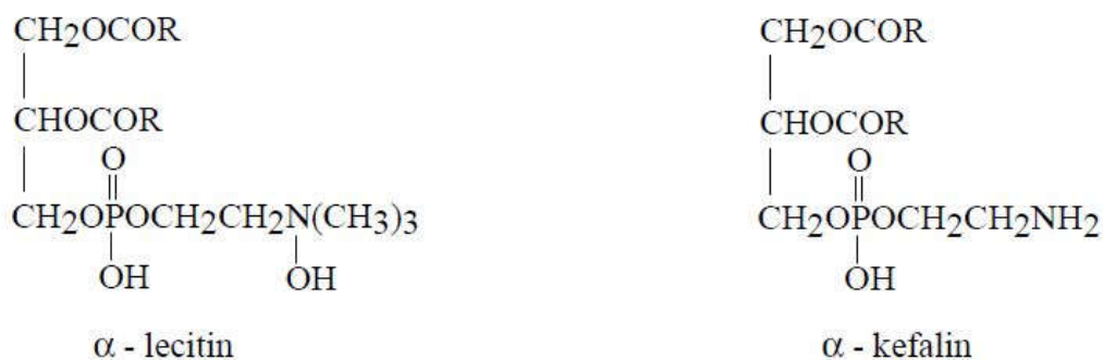
Slika 2 - Kemijska struktura negliceridnih sastojaka (Perinović-Jozić, 2003).
