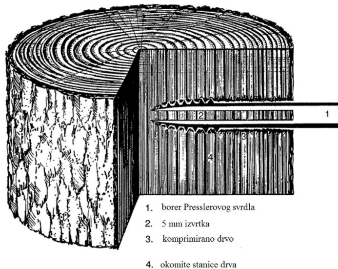
Slika 16. Shema ubušivanja borera Presslerovog svrdla u drvo (Speer, 2010)
