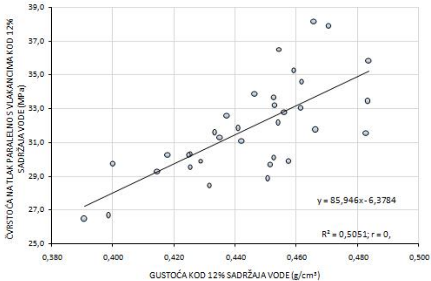
Slika 13. Graf ovisnosti čvrstoće na tlak paralelno s vlakancima o gustoći prirodne bijele topole kod 12% sadržaja vode
