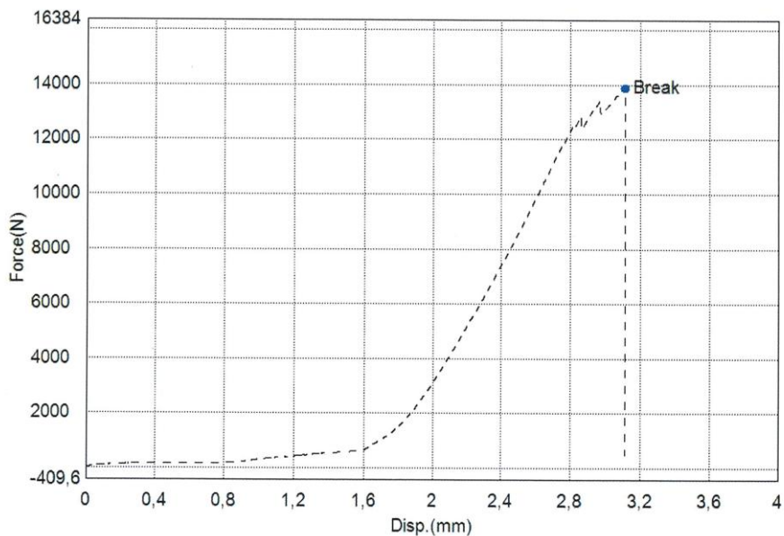
Slika 25. Tipičan grafički prikaz ispitivanja čvrstoće na vlak
