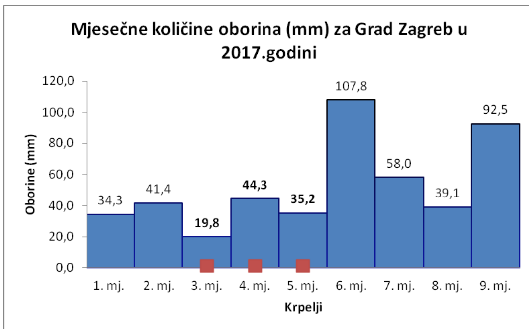
Slika 29. Grafički prikaz kretanja mjesečnih količina oborina za područje Grada Zagreba
