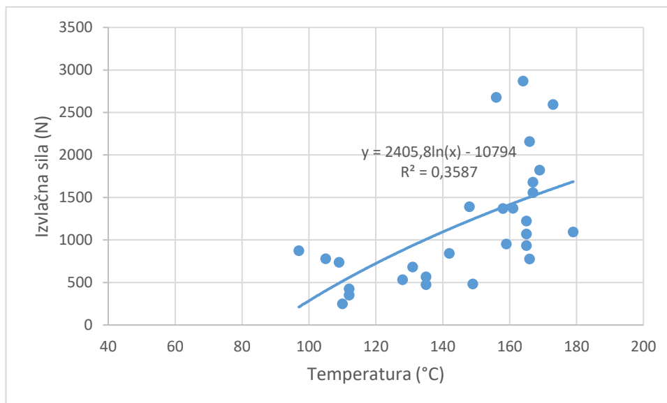
Graf 1. Utjecaj temperature na izvlačnu silu (BO_865_20)
