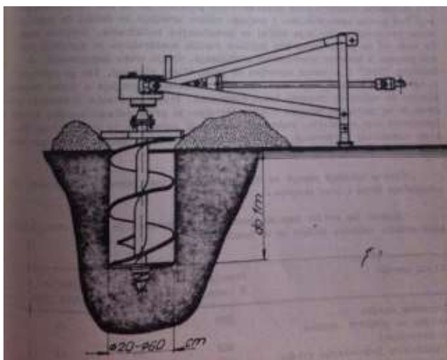
Slika 11. Bušilica Iva 1m
