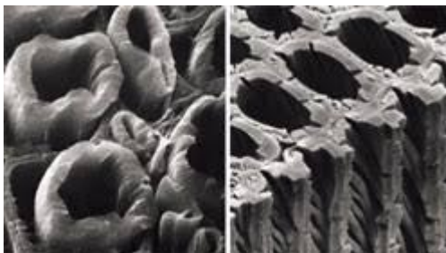
Slika 1. Anatomska građa: A) želatinoznih vlaknaca u drvu listača sa raslojavanjem staničnih stijenki, odnosno odstupanjem želatinskog sloja, i B) traheide kompresijskog drva sa značajnim helikalnim pukotinama (Preuzeto s https://korak.com.hr/korak-019-rujan-2007-reakcijsko-drvo/ )
