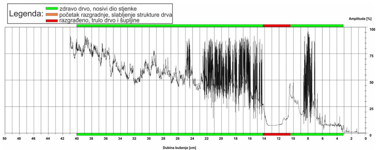
Slika 33: Rezistogram bušenja 15
