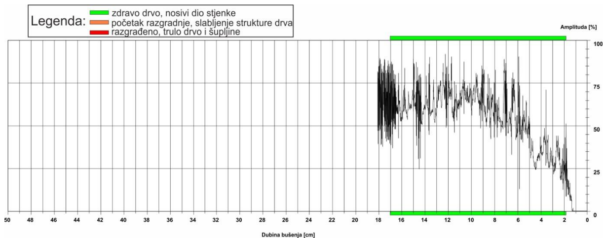
Slika 23: Rezistogram bušenja 8.1
