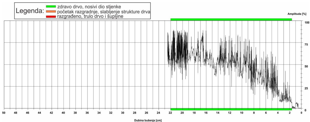
Slika 29: Rezistogram bušenja 12.1
