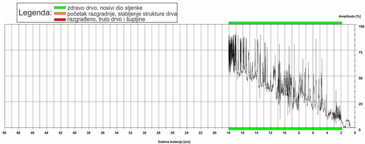
Slika 14: Rezistogram bušenja 1
