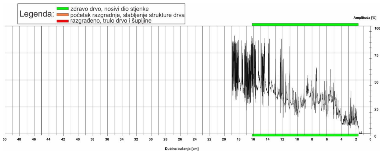
Slika 24: Rezistogram bušenja 9
