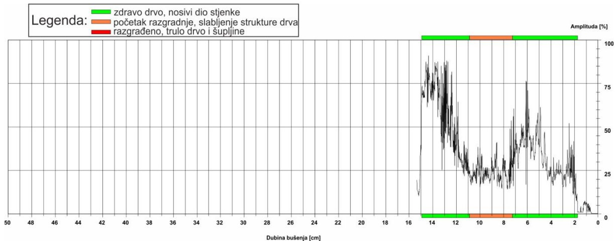
Slika 31: Rezistogram bušenja 13.1
