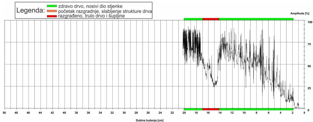
Slika 25: Rezistogram bušenja 10
