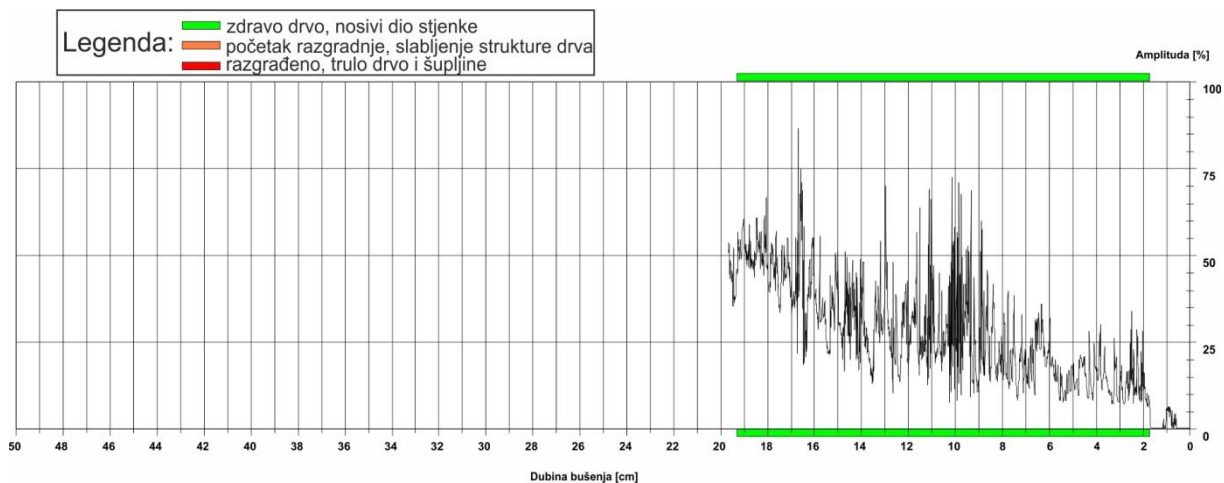
Slika 17: Rezistogram bušenja 5
