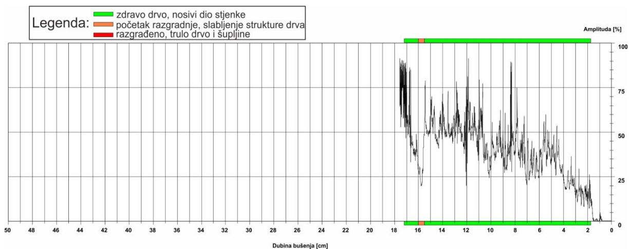
Slika 15: Rezistogram bušenja 2
