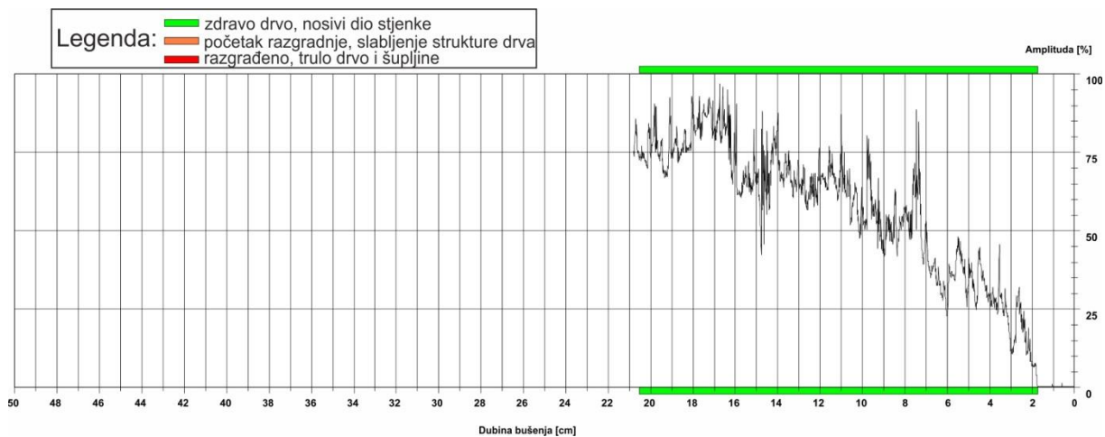
Slika 18: Rezistogram bušenja 5.1
