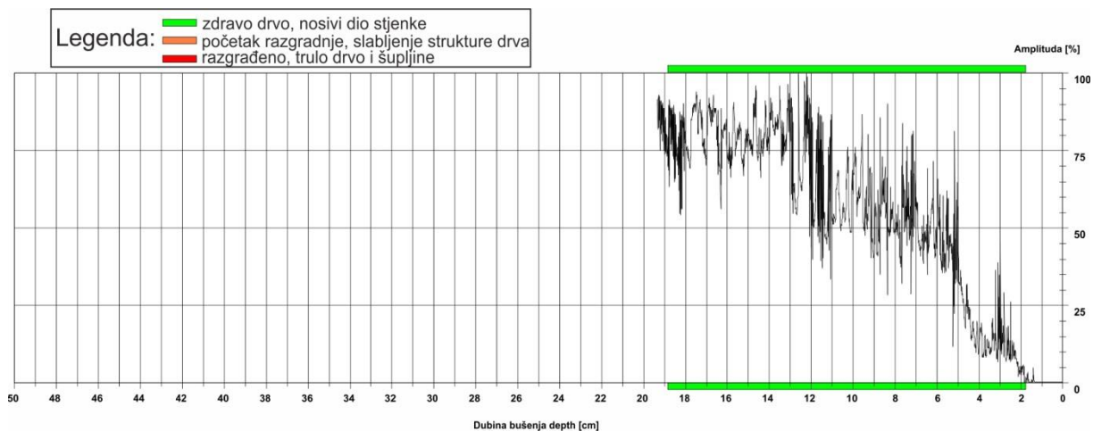
Slika 32: Rezistogram bušenja 14
