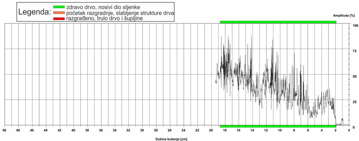
Slika 16: Rezistogram bušenja 3
