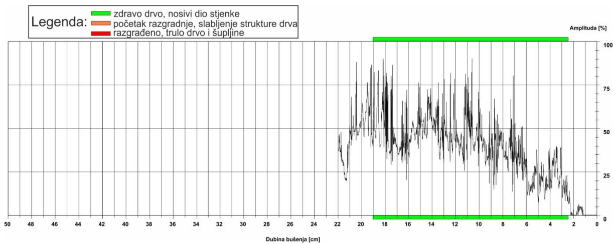
Slika 21: Rezistogram bušenja 6.1
