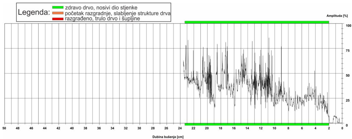
Slika 30: Rezistogram bušenja 13
