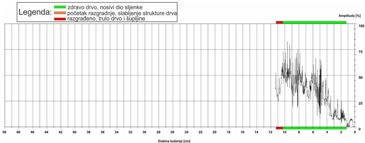
Slika 19: Rezistogram bušenja 7
