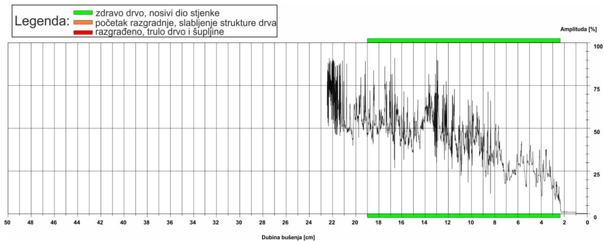
Slika 20: Rezistogram bušenja 6
