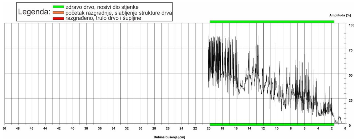
Slika 22: Rezistogram bušenja 8
