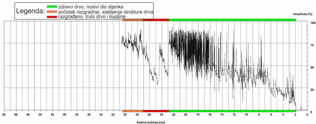
Slika 26: Rezistogram bušenja 11
