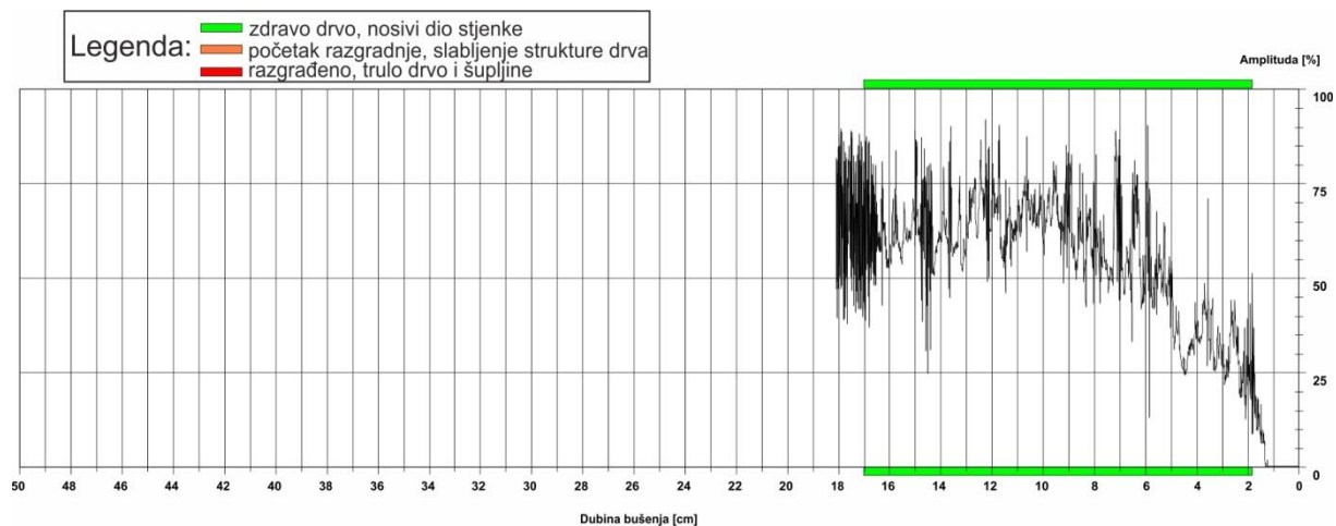
Slika 23: Rezistogram bušenja 8.1
