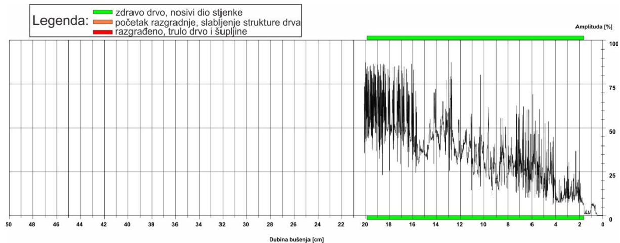
Slika 22: Rezistogram bušenja 8
