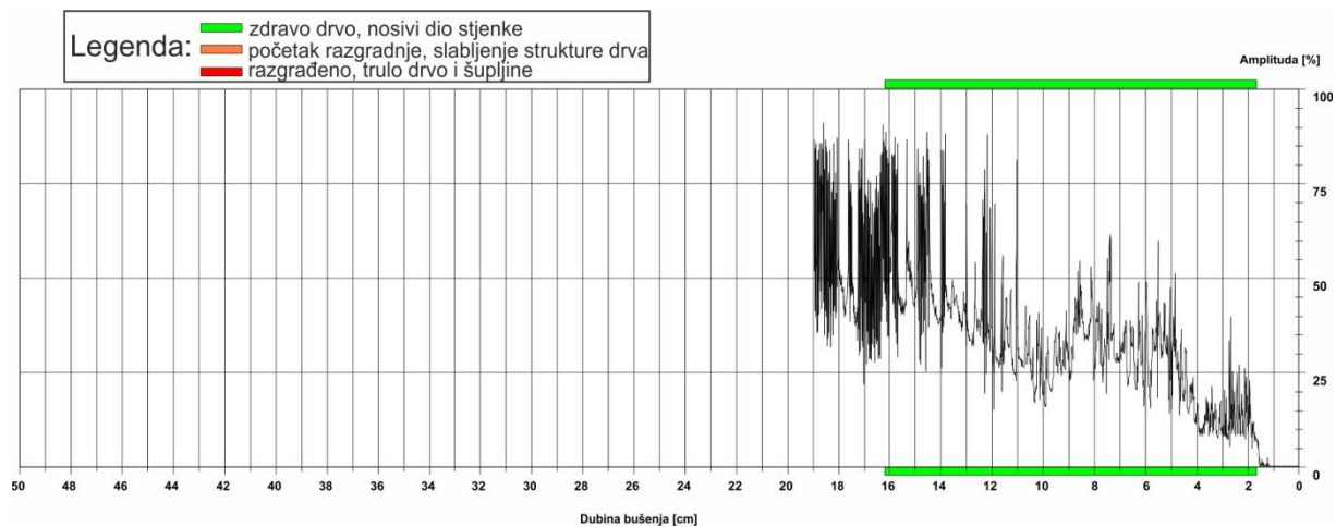
Slika 24: Rezistogram bušenja 9
