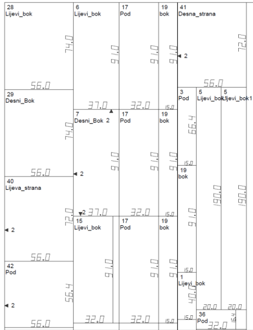
Slika 21. Shema krojenja panela 1 izradena softverom Panel Wizard
