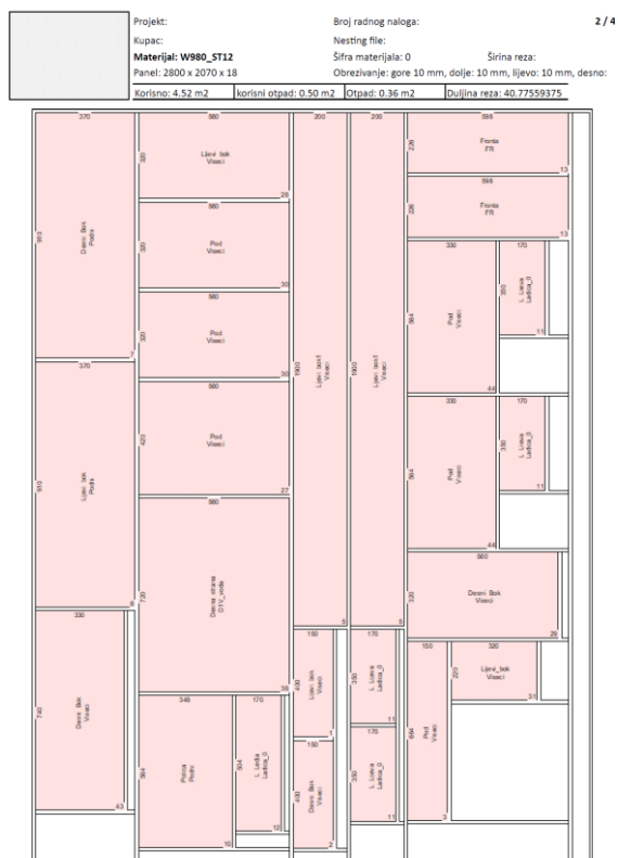
Slika 27. Shema 3 krojenja svih elemenata izrađena softverom Corpus
