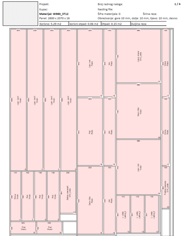
Slika 25. Shema 1 krojenja svih elemenata izradena softverom Corpus
