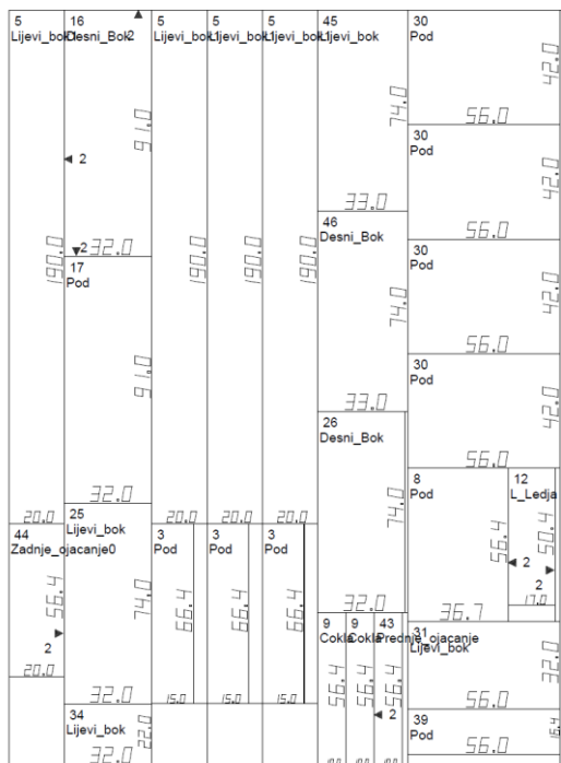
Slika 22. Shema 2 krojenja svih elemenata izradena softverom Panel Wizard
