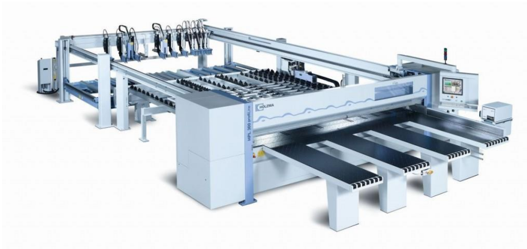
Slika 5. Horizontalni raskrajač
