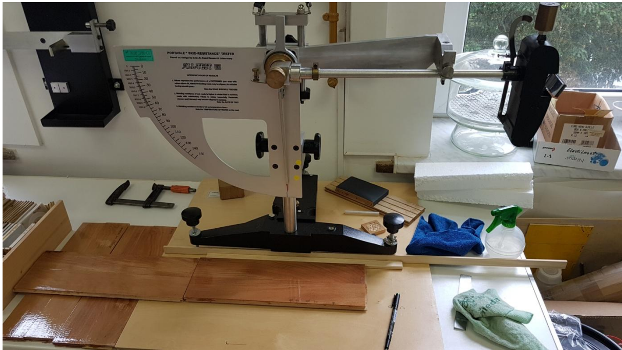
Slika 19. Njihalo za ispitivanje klizavosti
