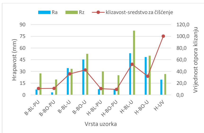
Slika 51. Utjecaj hrapavosti površine na klizavost navlažene površine sa sredstvom za čišćenje
